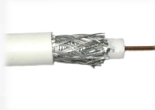
PRZEWÓD KONCENTRYCZNY
